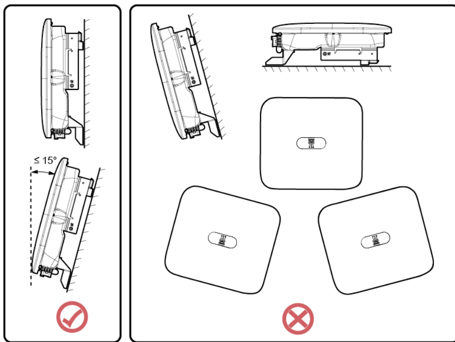
Figura 4-1 Posición de instalación
