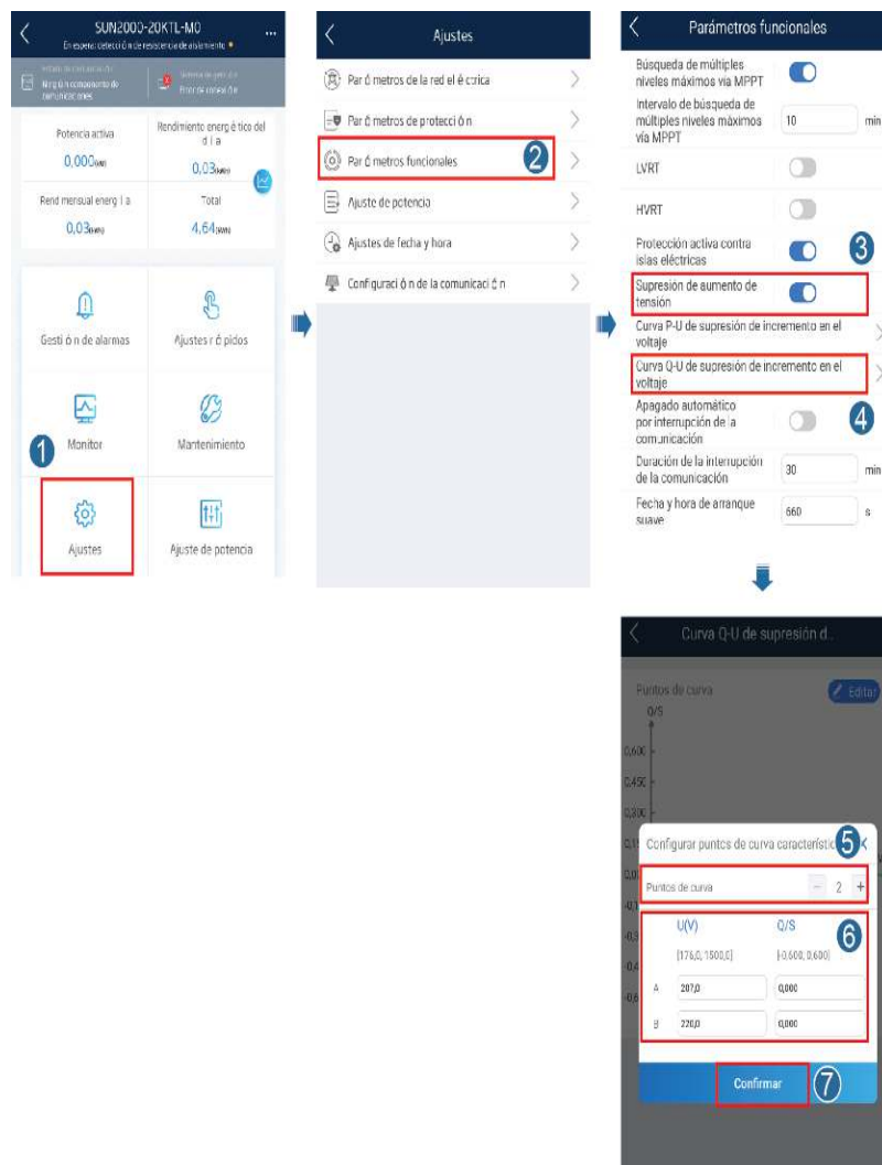
Figura D-1 Configuración de los parámetros de la curva Q-U de supresión de incremento en la tensión
