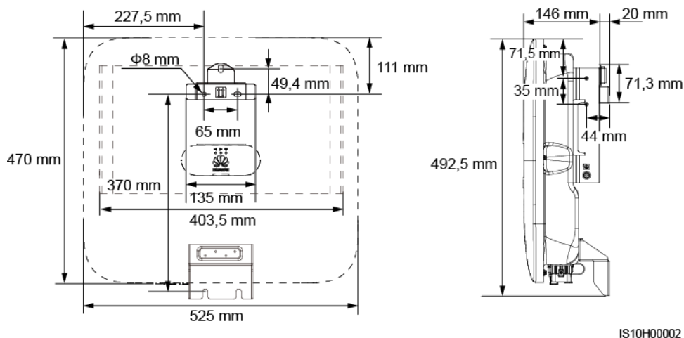
Figura 4-6 Dimensiones de la ménsula de montaje
