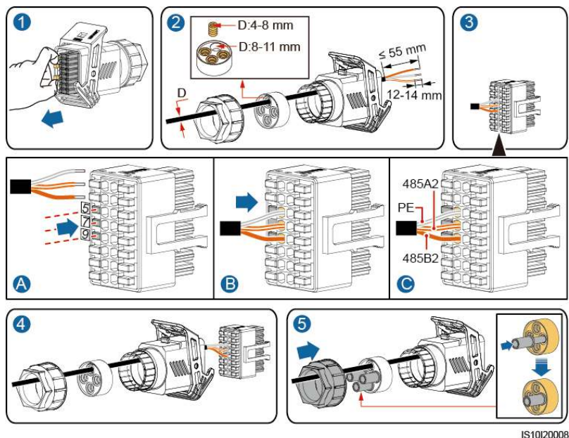
Figura 5-26 Cómo instalar el cable
