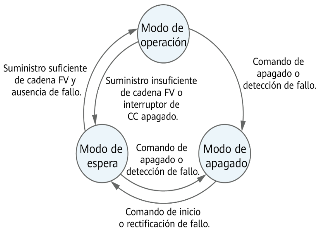
Figura 2-8 modos de operación
