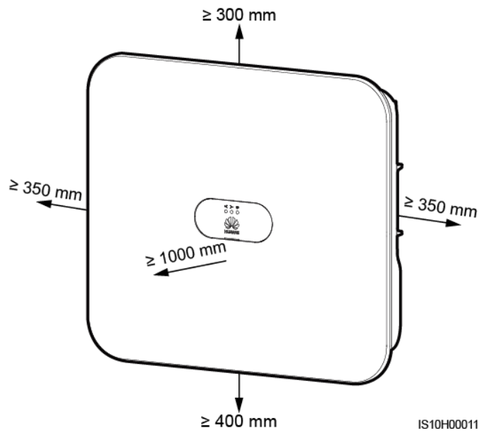
Figura 4-2 Espacio de instalación
