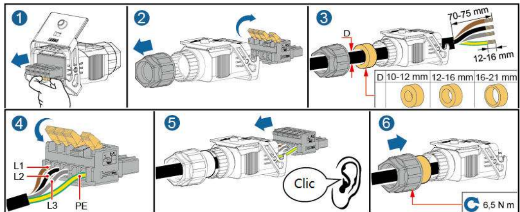
Figura 5-6 Cable de cuatro conductores (L1, L2, L3 y conexión a tierra)
