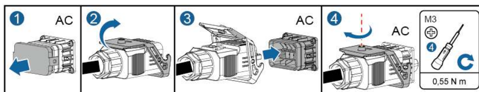
Figura 5-9 Cómo fijar el conector de CA
